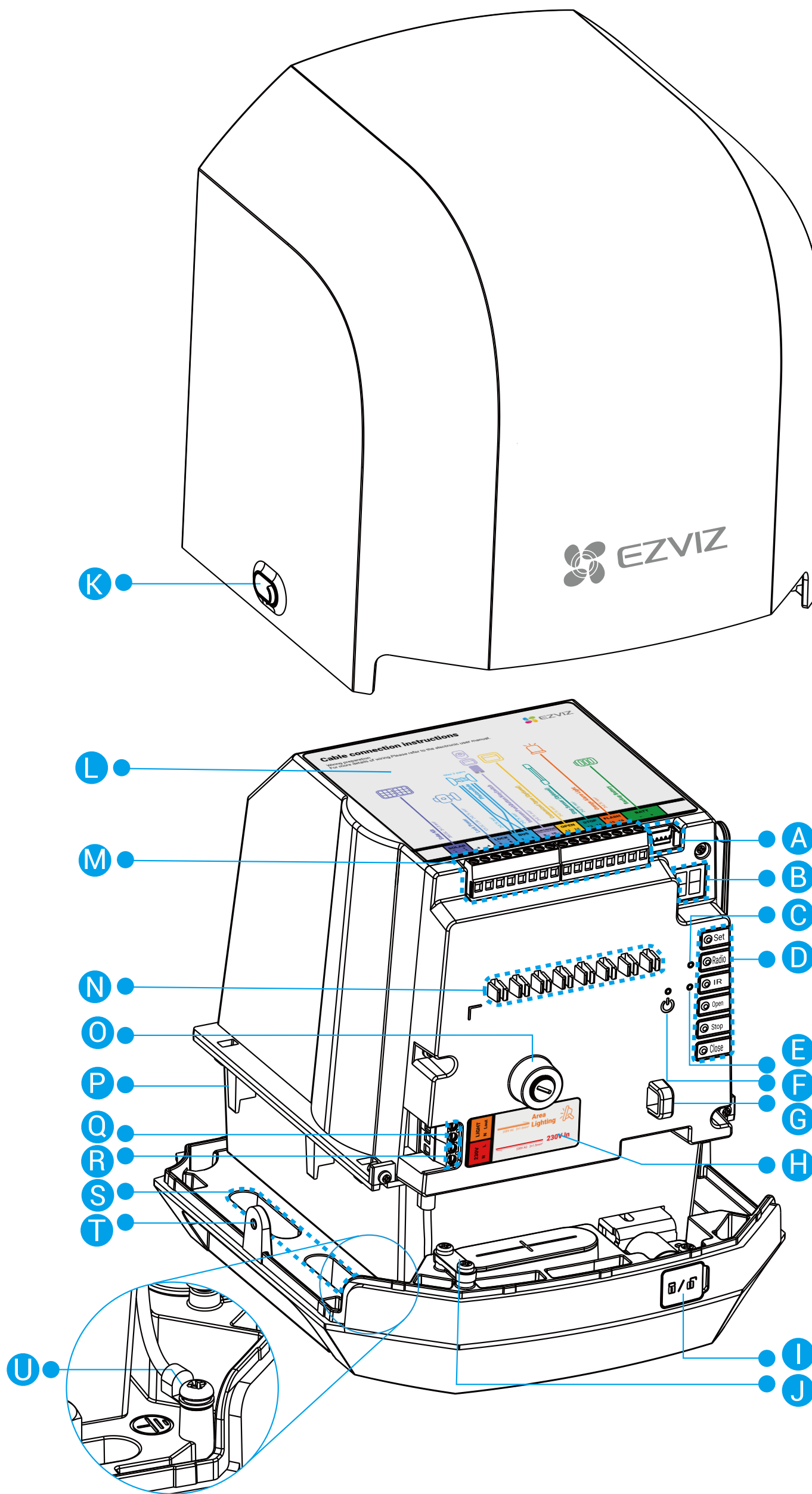
Přední pohled
